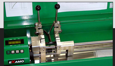
Zugtest mit dem Leister EXAMO USB
