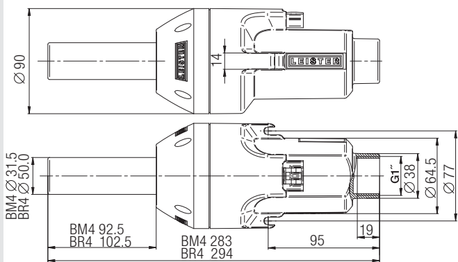
Einbau schematisch
