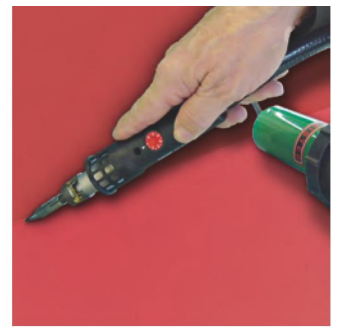
LABOR S gekoppelt mit dem MINOR als externe Luftversorgung.
